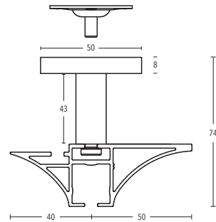
Ceiling bracket 43 mm and 73 mm Art. no. 11473-50 und 11473-80
